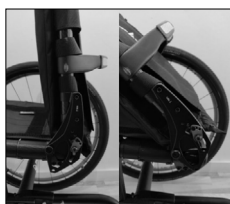
APBC20 Nedfällbar rygg med lås (standard)
